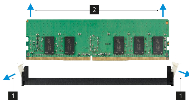
Рис. 27. Извлечение модуля ОЗУ
