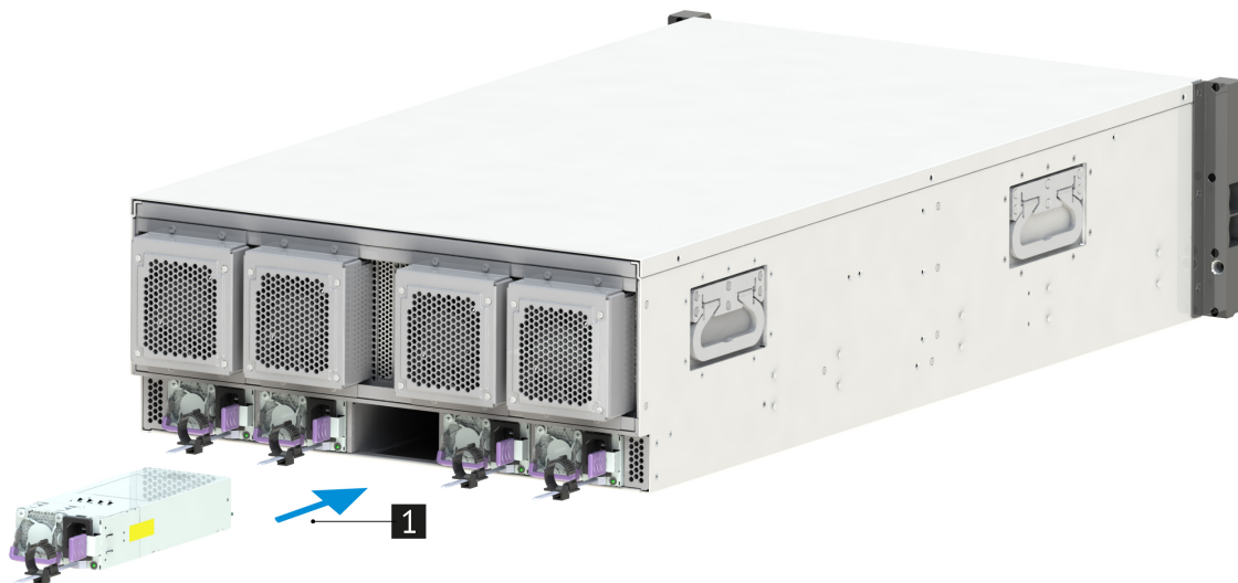
Рис. 52. Установка блока питания сервера
