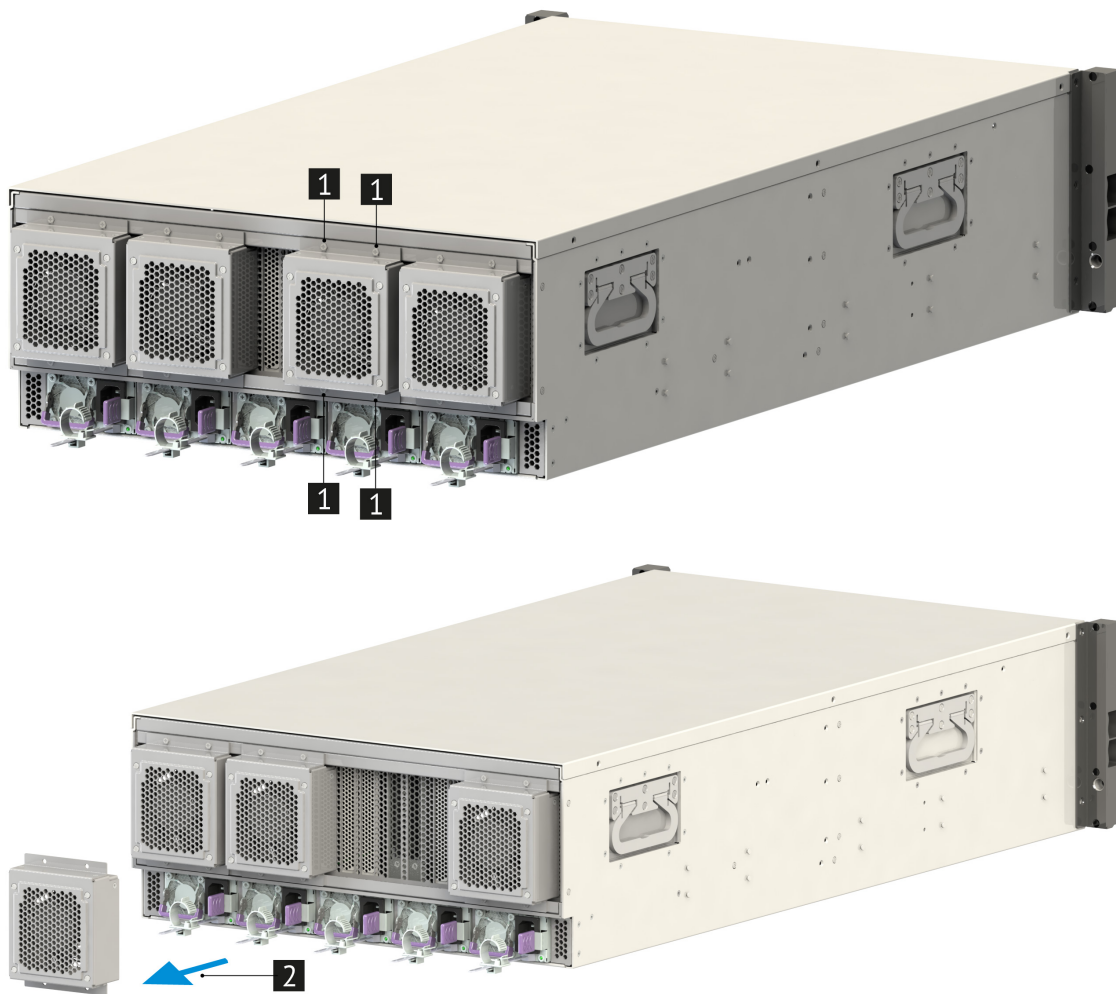
Рис. 24. Извлечение наружного вентилятора сервера
