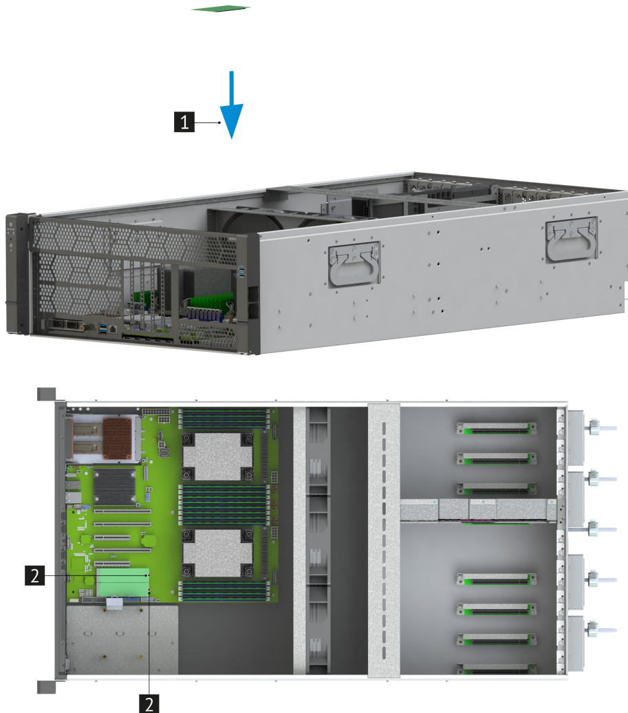
Рис. 35. Установка M.2 диска
