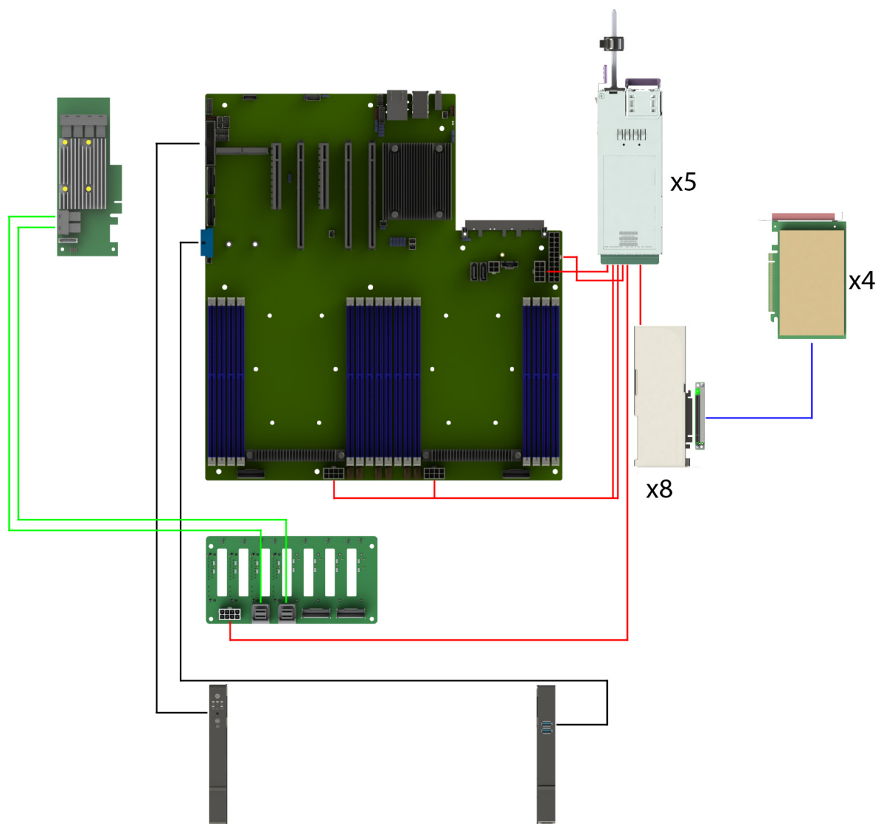
Рис. 21. Схема прокладки системных кабелей, кабелей питания, кабелей для подключения дисков SAS/SATA с подключением PCIe RAID
