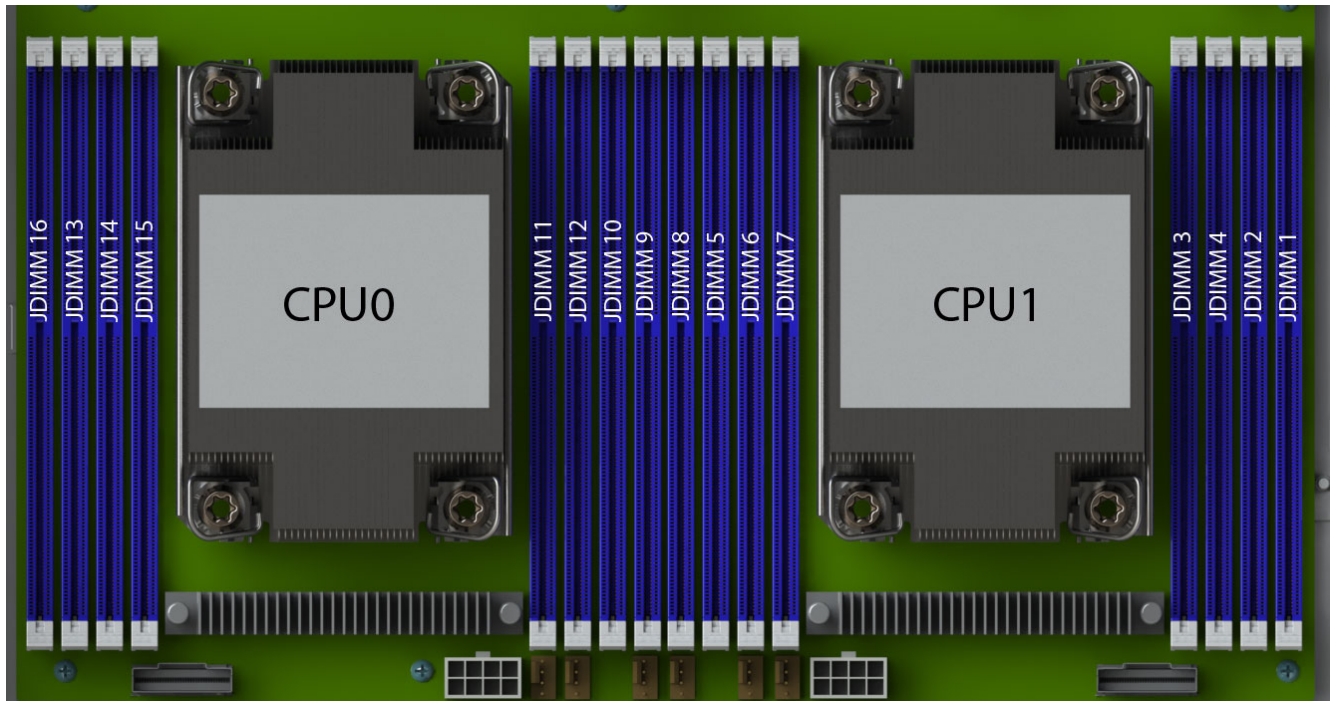
Рис. 26. Расположение разъемов
