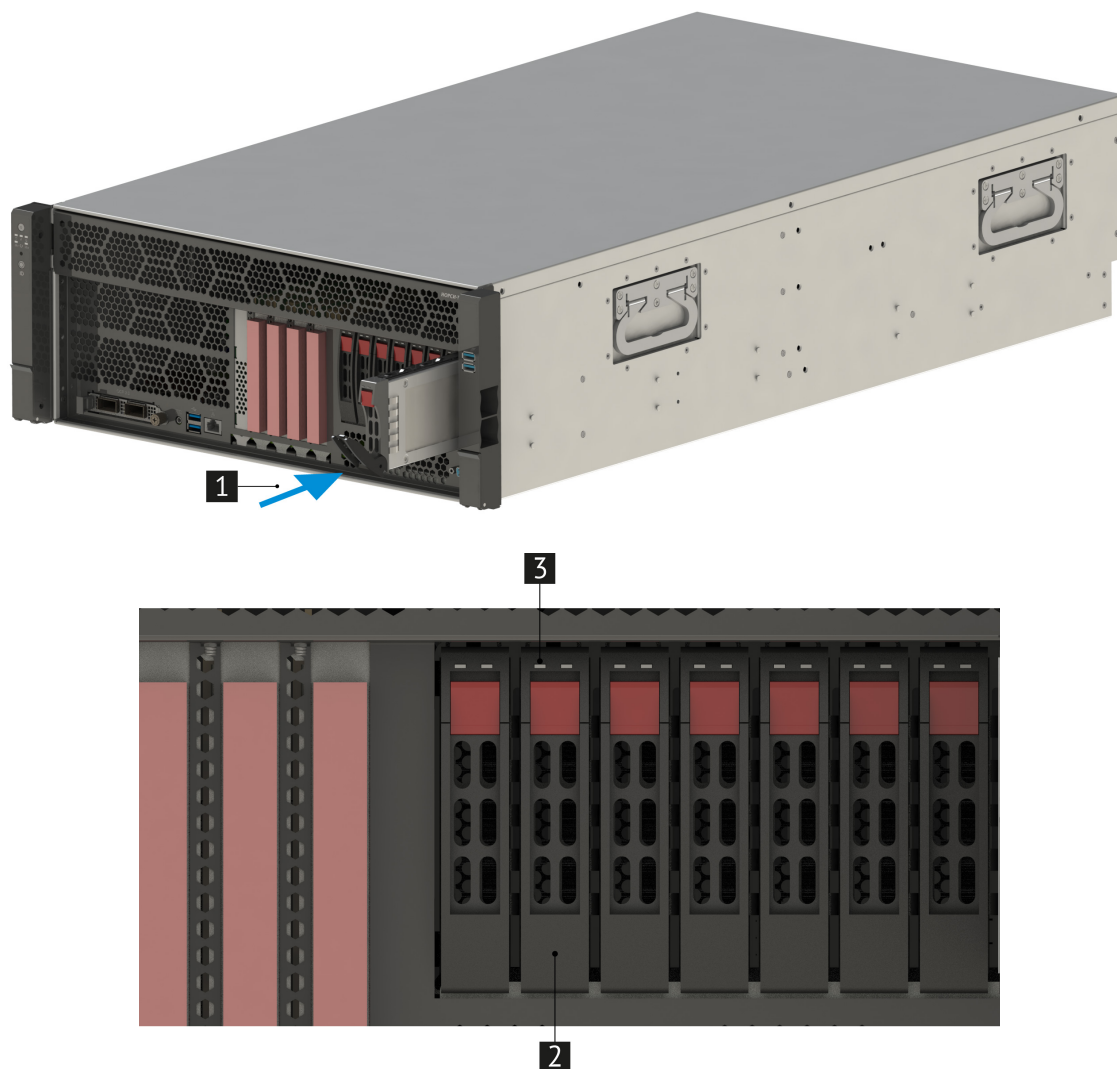
Рис. 39. Установка дисков
