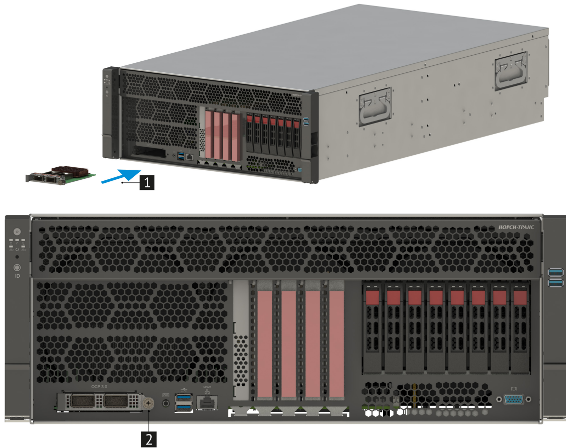
Рис. 45. Установка карты OCP 3.0 PCIe x16
