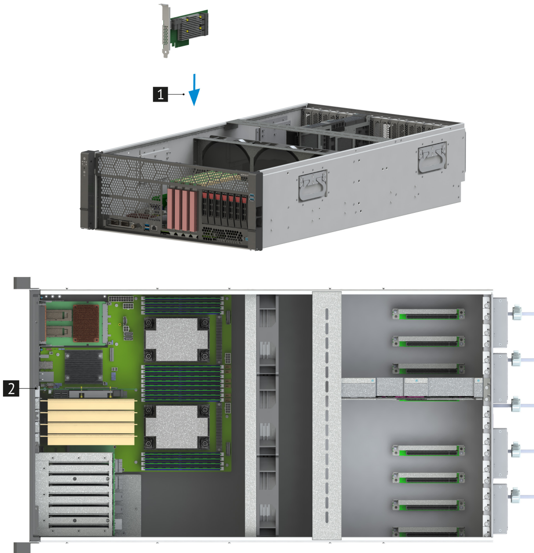
Рис. 41. Установка SAS3 12G RAID-контроллер 24I
