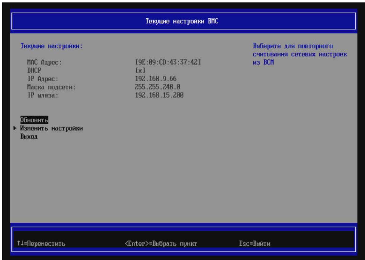
Рис. 59. Меню «Текущие настройки ВМС»
