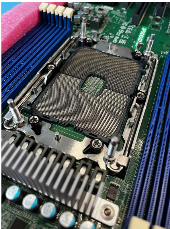
Рис. 30. Снятие модуля процессора с радиатором
