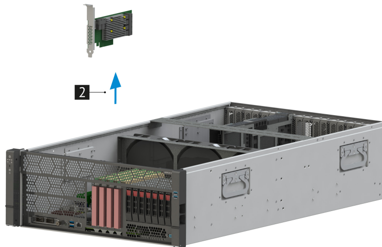
Рис. 40. Извлечение SAS3 12G RAID-контроллера 24I
