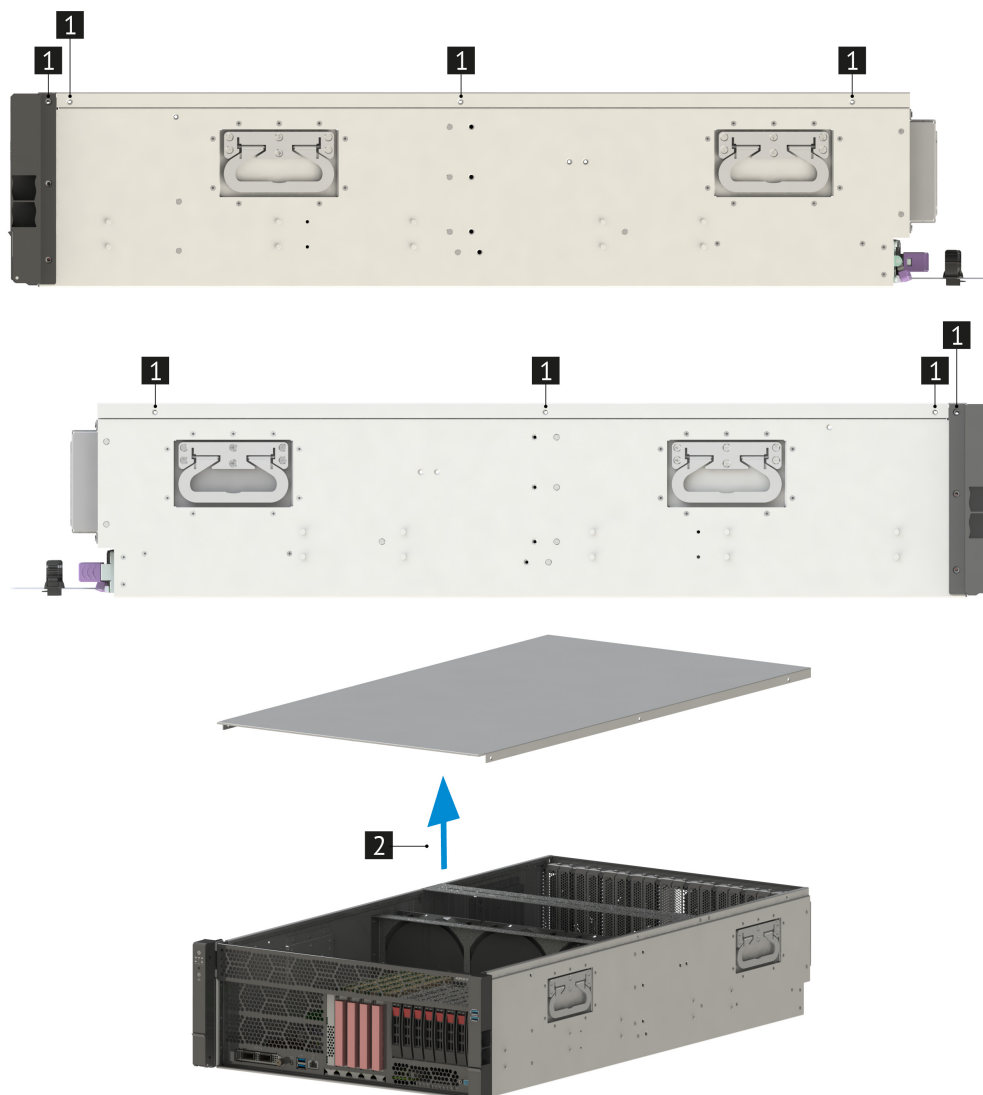
Рис. 13. Снятие верхней крышки платформы
