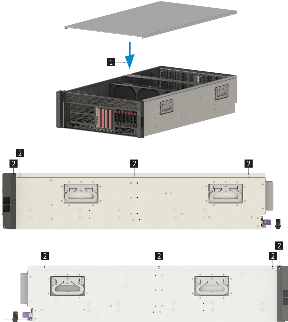
Рис. 14. Установка верхней крышки платформы
