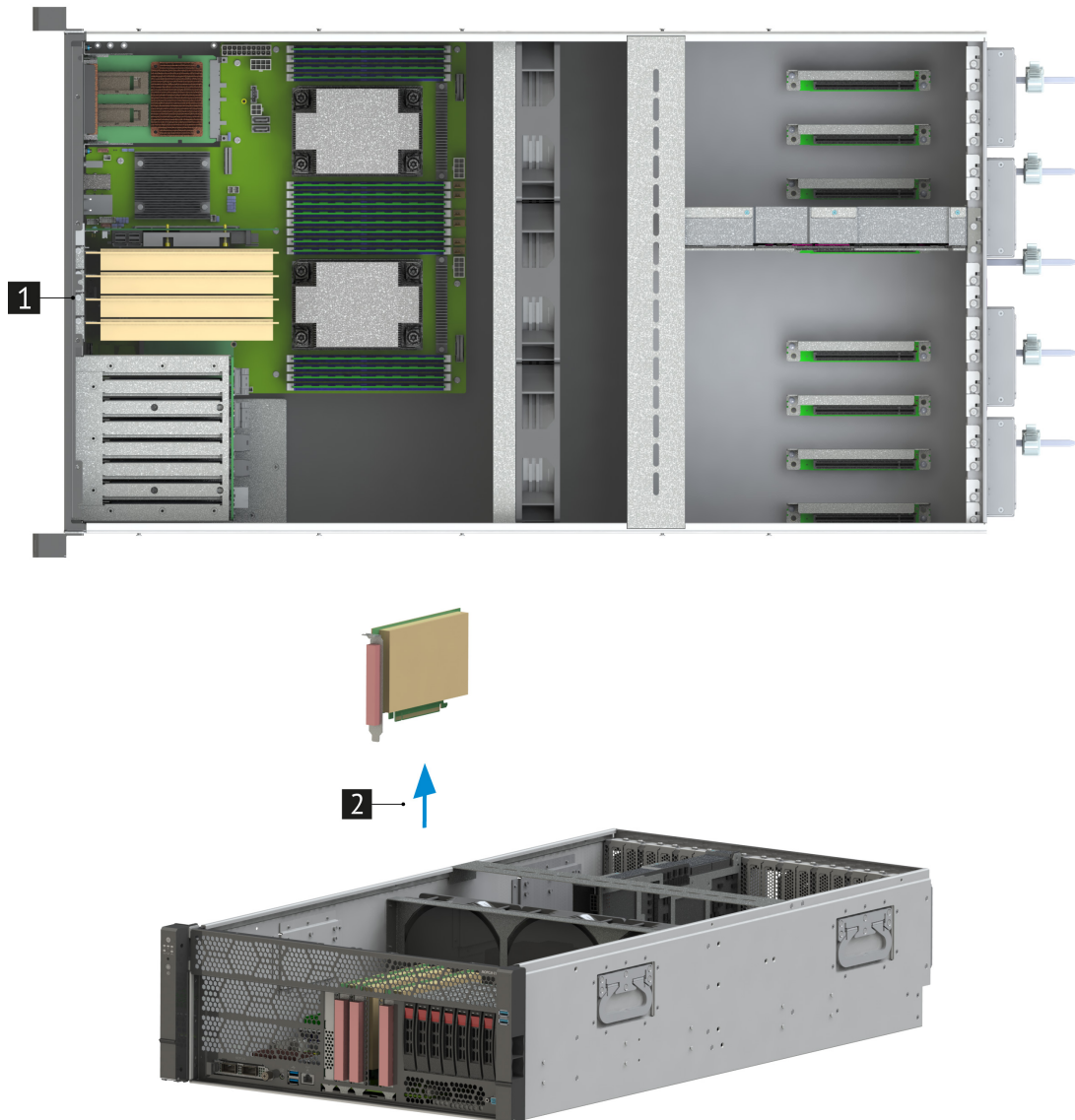
Рис. 42. Извлечение карты PCIe
