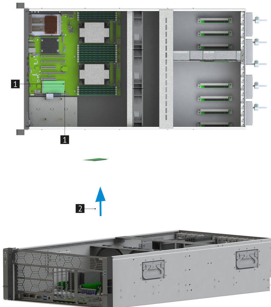
Рис. 34. Извлечение М.2 диска
