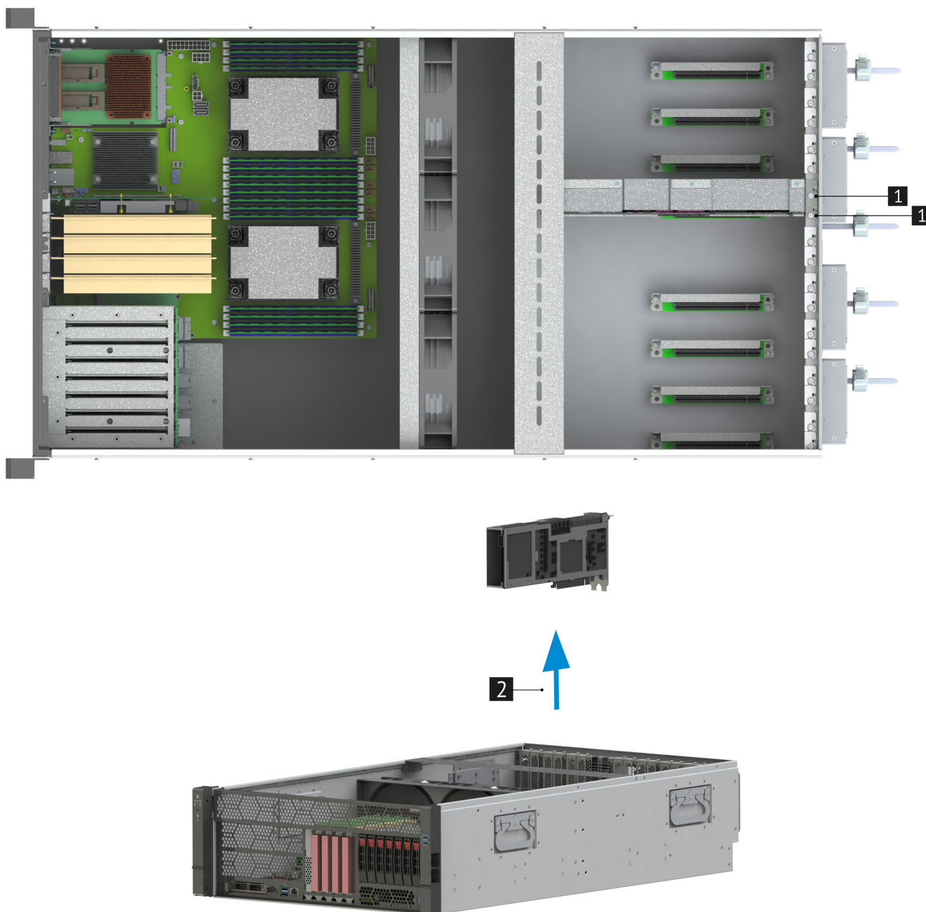
Рис. 46. Извлечение карты GPU
