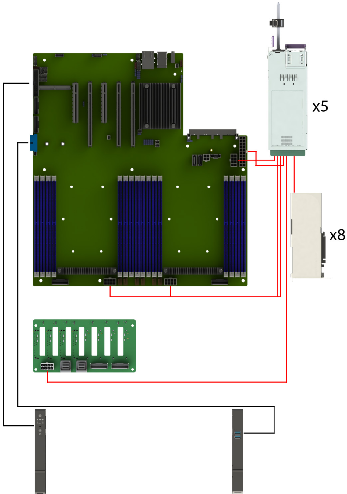
Рис. 18. Схема прокладки системных кабелей и кабелей питания
