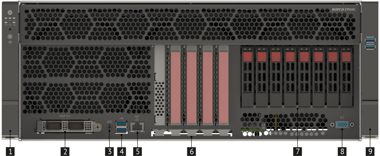
Рис. 2. Вид сервера спереди с 8-ю установленными жесткими дисками
