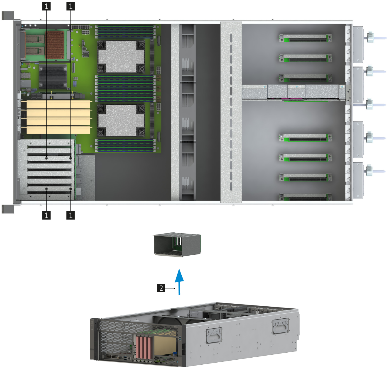
Рис. 15. Извлечение каркаса под диски SFF
