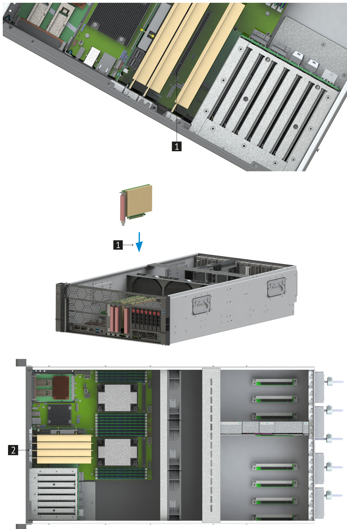
Рис. 43. Установка карты PCIe
