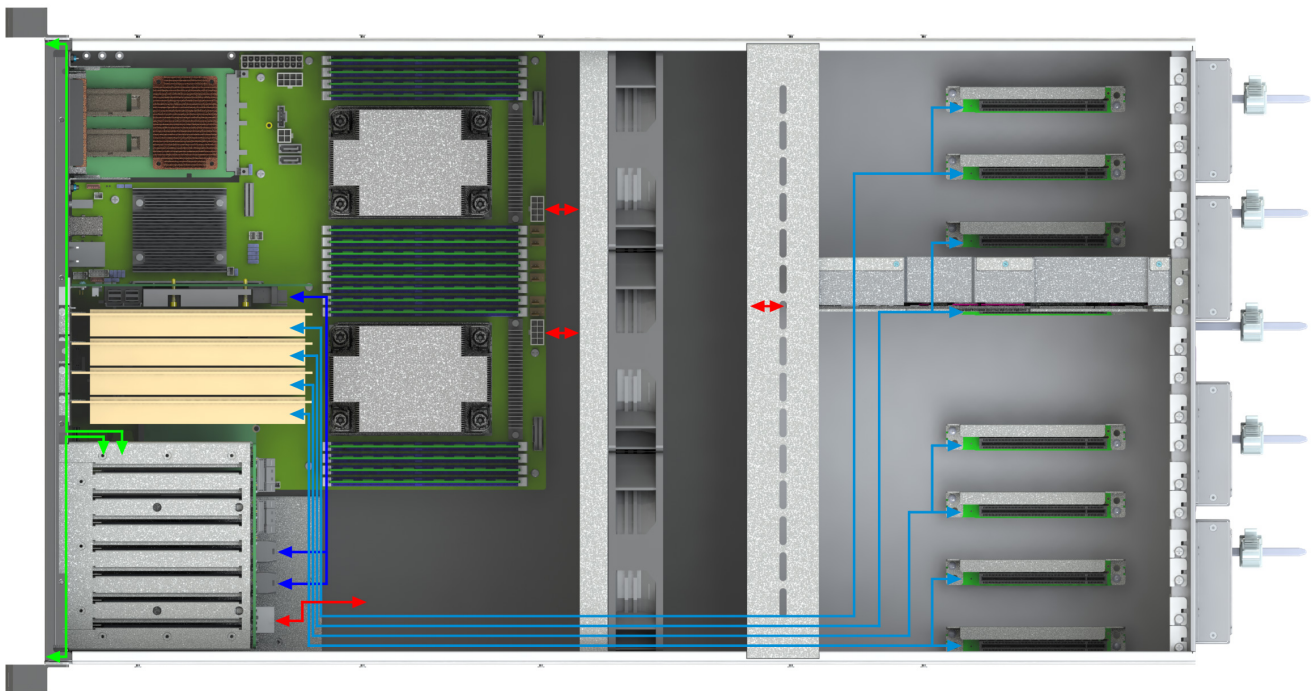
Рис. 17. Схема прокладки кабелей в сервере
