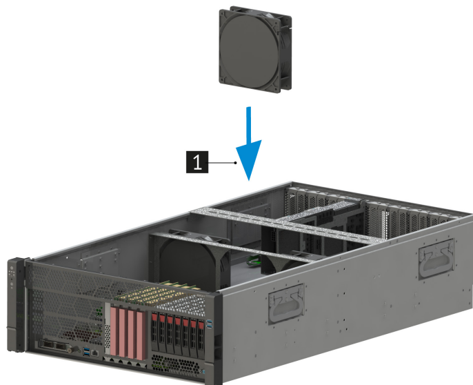
Рис. 23. Подключение вентилятора
