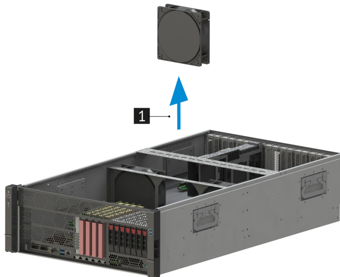
Рис. 22. Извлечение вентилятора из сервера
