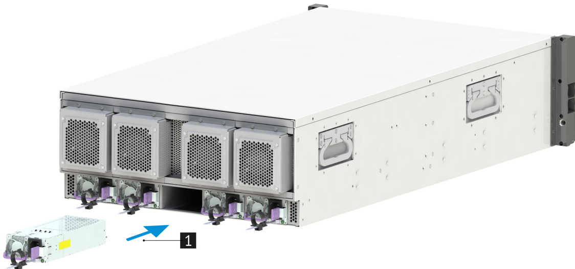
Рис. 50. Установка блока питания в сервер
