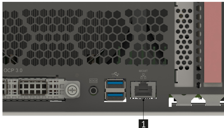
Рис. 6. Сетевые интерфейсы
