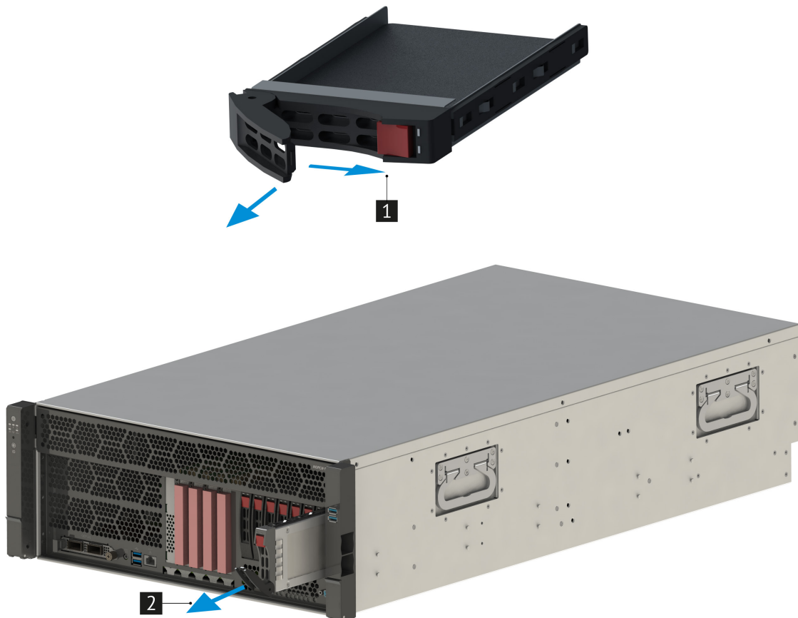
Рис. 38. Извлечение дисков
