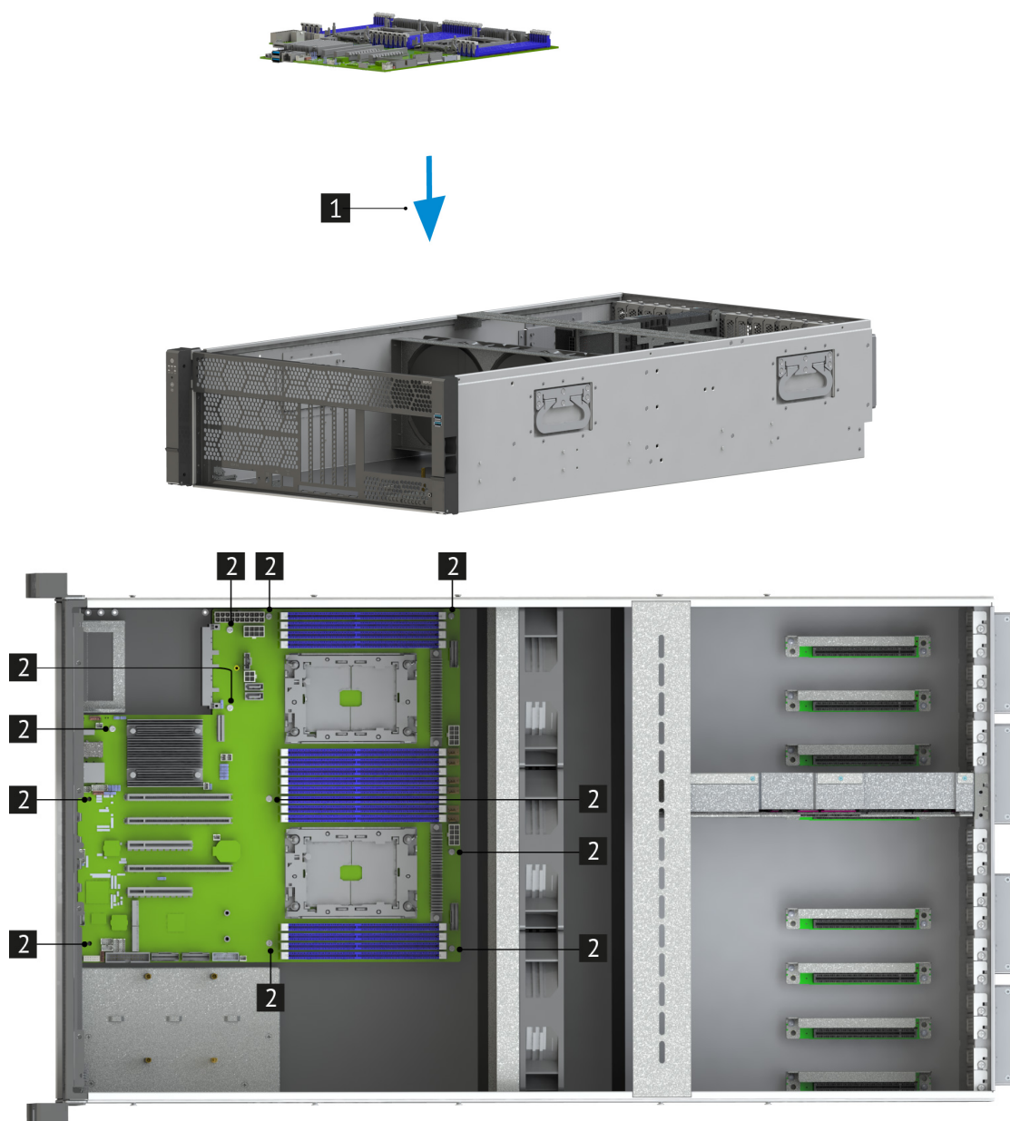
Рис. 37. Установка материнской платы в сервер
