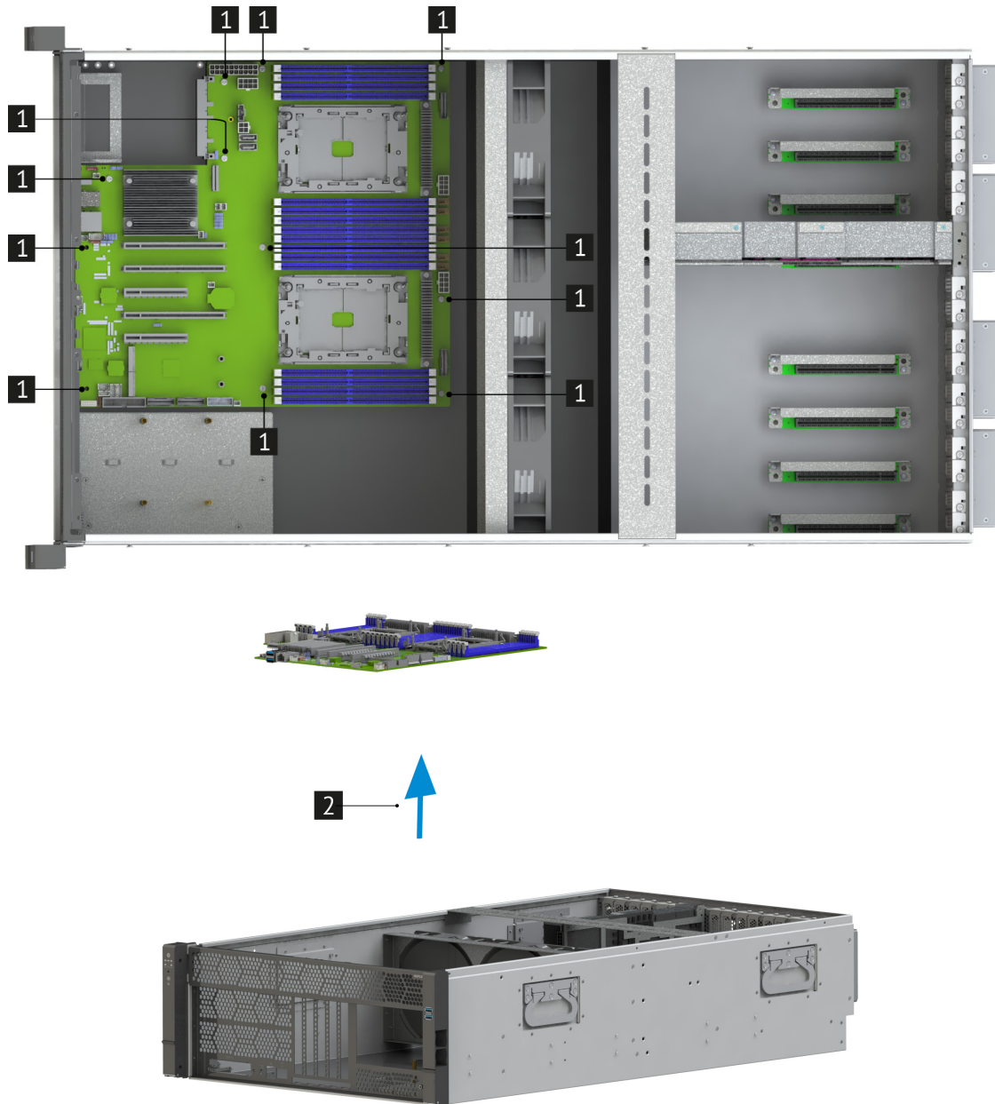
Рис. 36. Извлечение материнской платы из сервера
